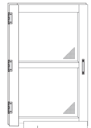
枠なし開き網戸 （丁番、取手、マグネット付き） P73
