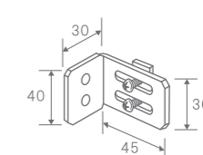
No.041-L ※L金具
