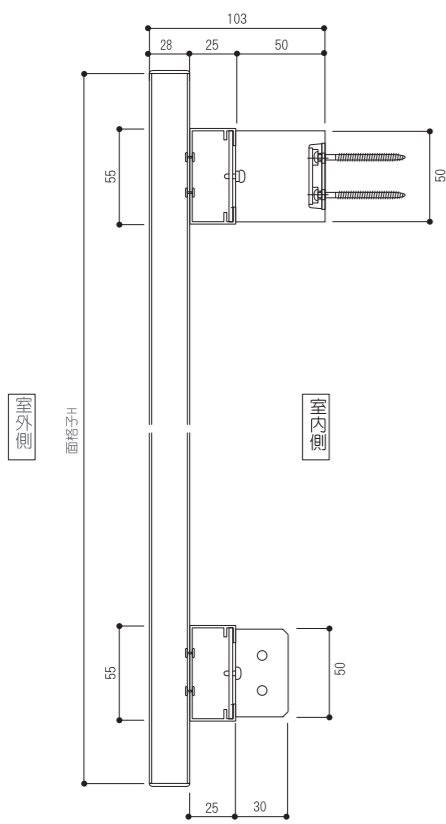
■縦断面図
