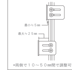
■L金具の可動範囲(面格子側)
