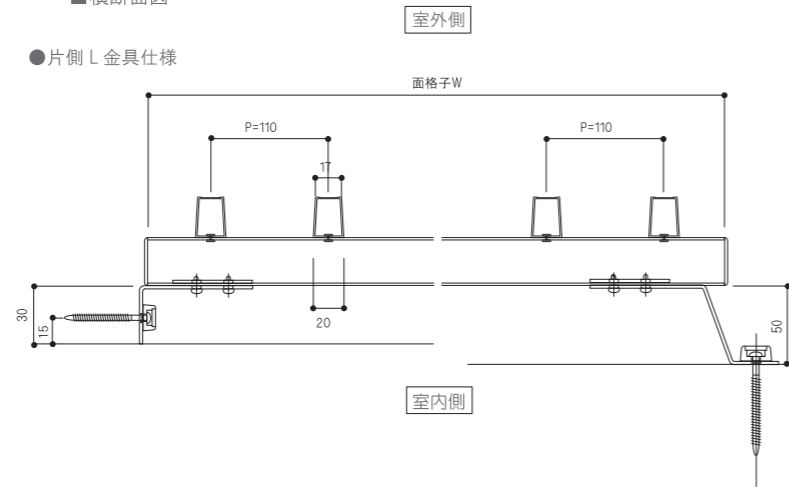
■横断面図
