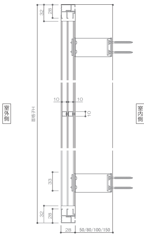
■縦断面図
