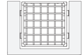
■格子出来寸法 開口W=20mm/開口H=10mm
