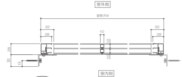
■横断面図
