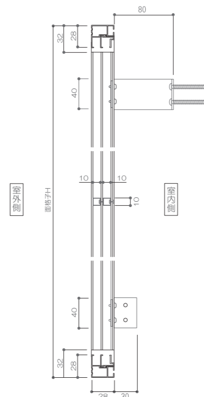
■縦断面図
