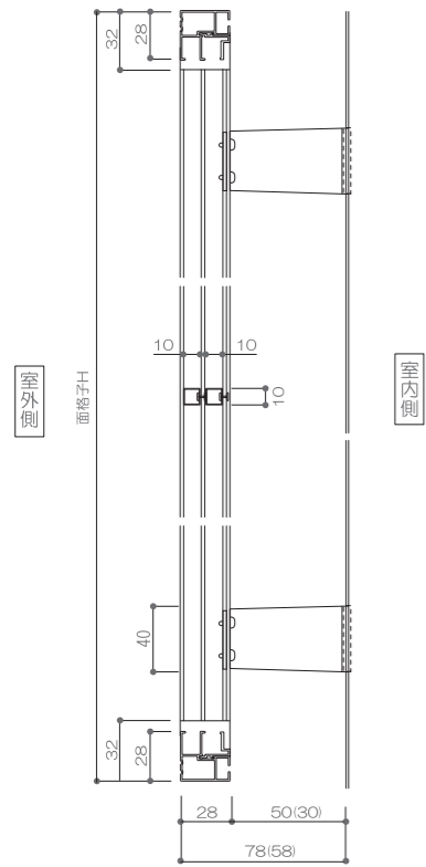
■縦断面図
