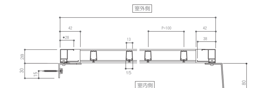
■横断面図
