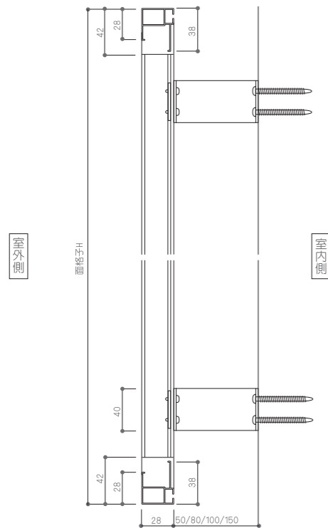
■縦断面図
