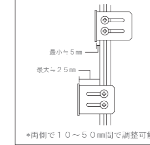
■L金具の可動範囲 (面格子側)
