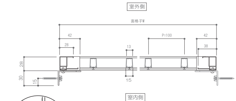
■横断面図
