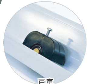
戸車 上部より調節ができます。
