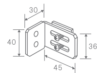
No.031-L L金具
