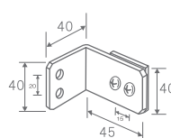
No.011 ※L金具
