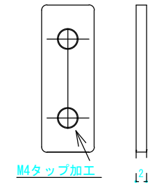
枠付き格子用 座金
