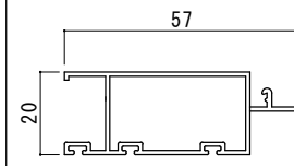
ビル用縦框
