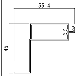
ビル用縦框
