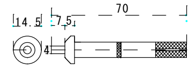
格子取付ホールインアンカー
