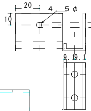
座金防止金具
