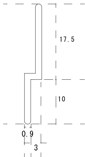
薄型Sレール
