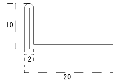
ステン土間レール
