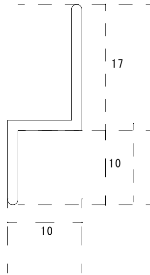
Sレール
