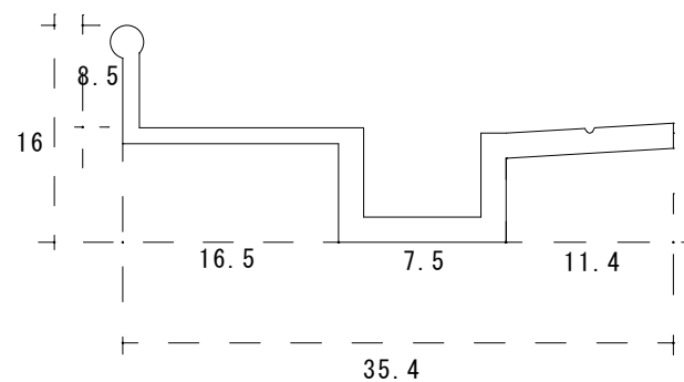
袋型用持ち出しレール
