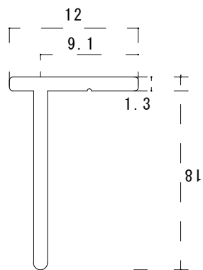
木製建具用Tレール
