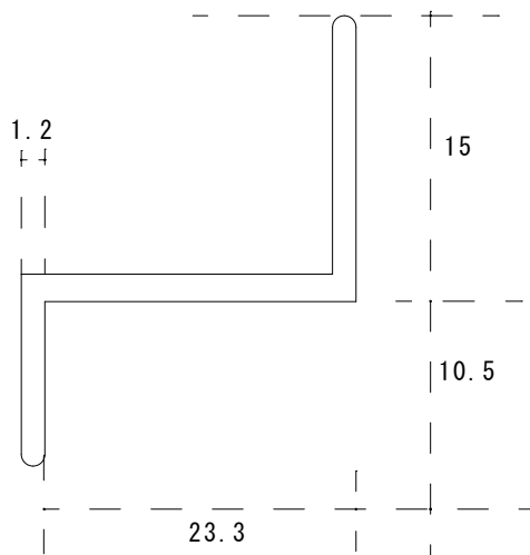
袋型用クランクレール
