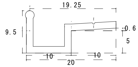
持出レール
